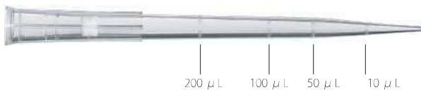
0.5-200 \mu L ロング フィルター付き 滅菌済 77.5 mm
